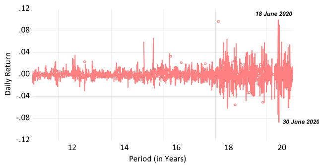
Figure 7 Ln return (sugarcane)
